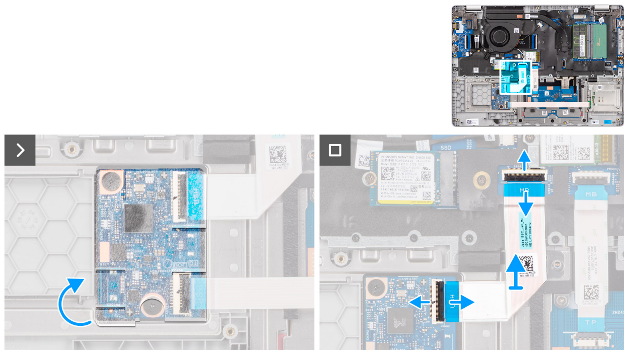
Figure 35. Retrait du FPC de la carte USH
