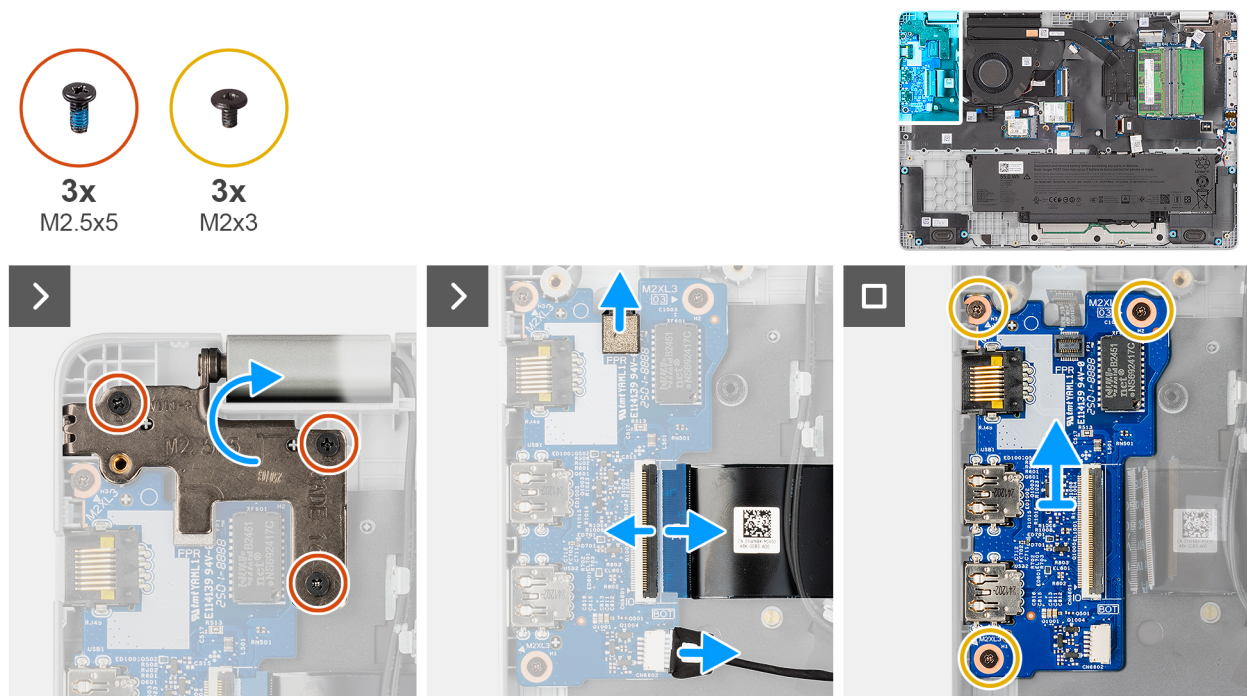
Figure 51. Retrait de la carte d'E/S
